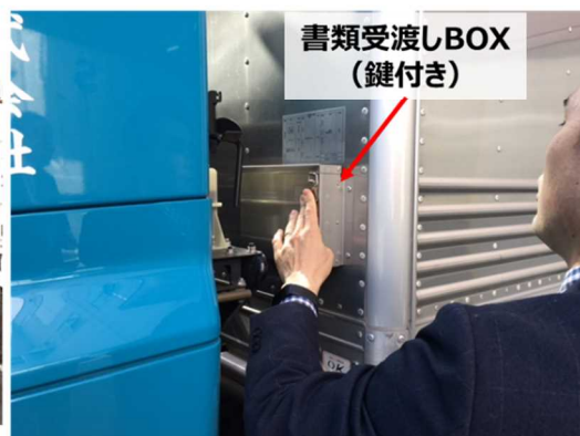
図表4-2-3 脱着ボディコンテナ
